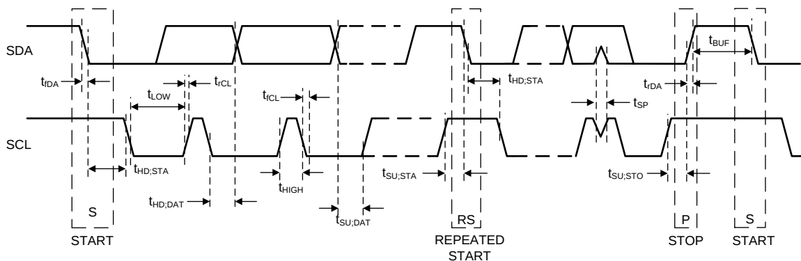
图 24. I²C-Compatible Timing
