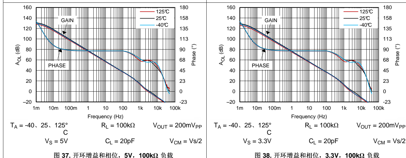
图 37. 开环增益和相位, 5V, 100kΩ 负载
