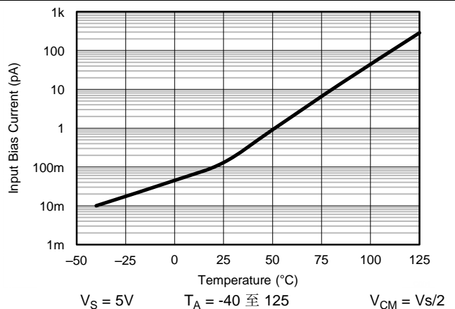
图 14. 输入偏置电流与温度间的关系
