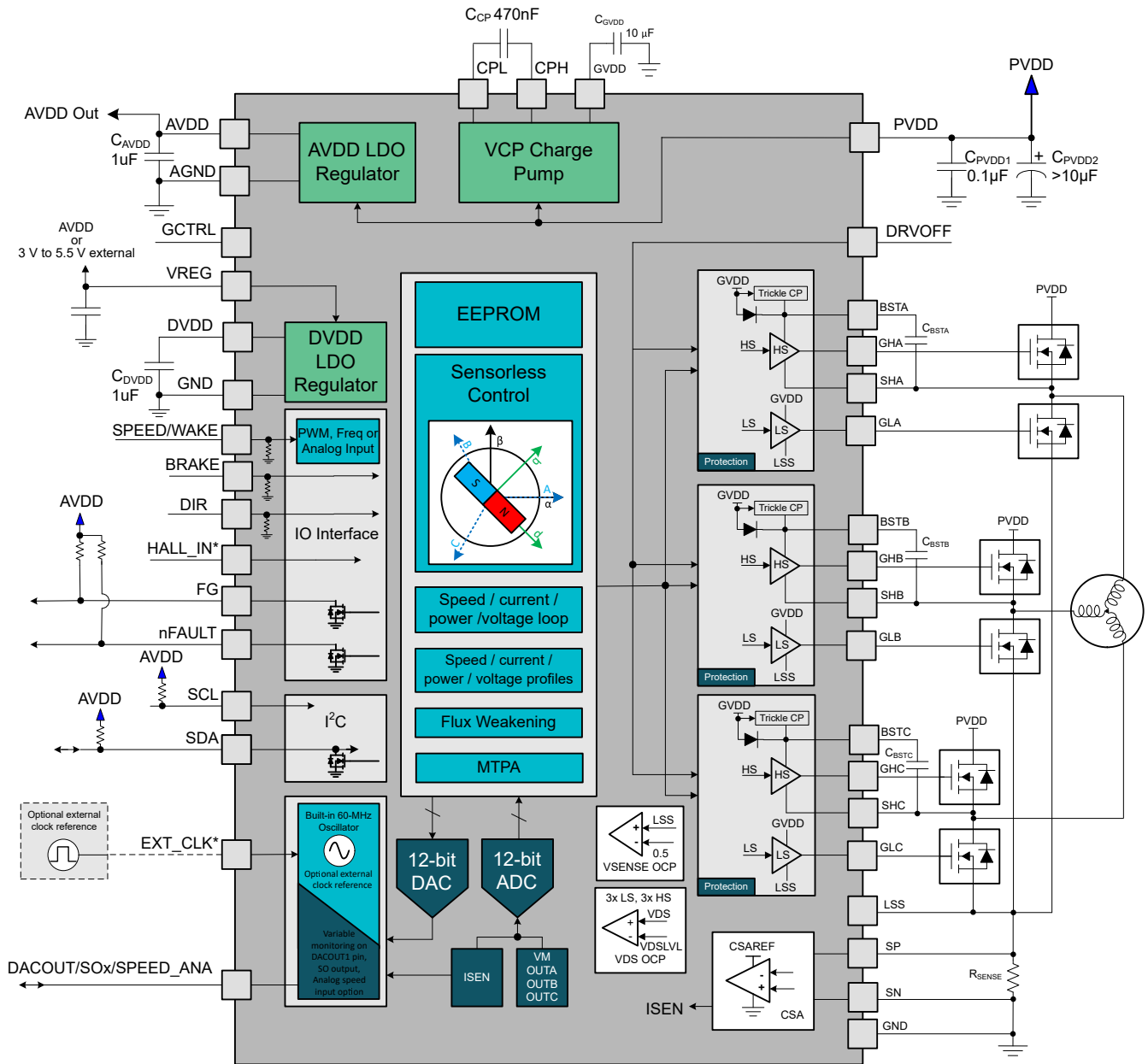
图 7-1. MCF8329HS 功能方框图
