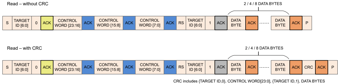
图 7-56. I 2 C 读取事务序列
