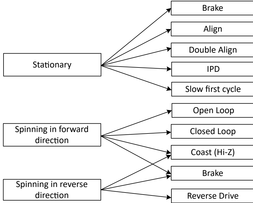
图 7-21. 在不同初始条件下启动电机
