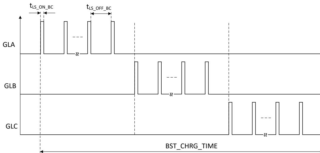
图 7-20. 启动时对自举电容器进行预充电
