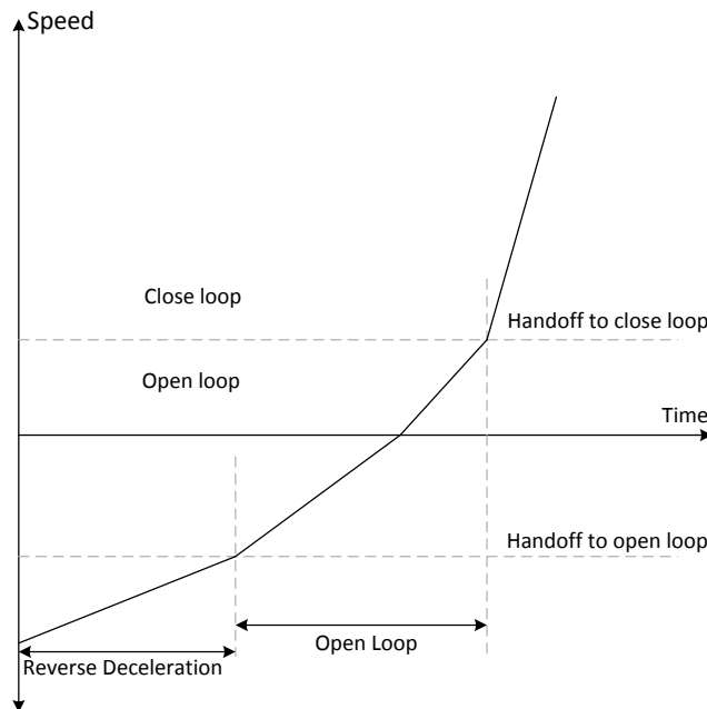
图 7-23. 反向驱动功能
