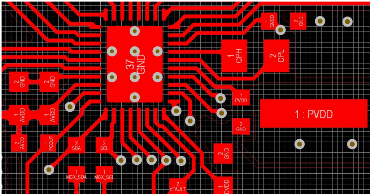
图 10-7. MCF8329HS 器件布局示例
