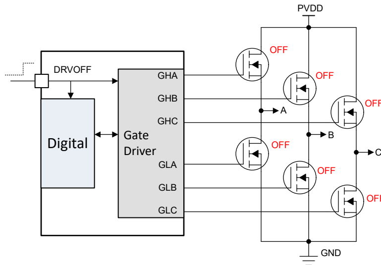
图 7-52. DRVOFF 栅极驱动器输出状态
