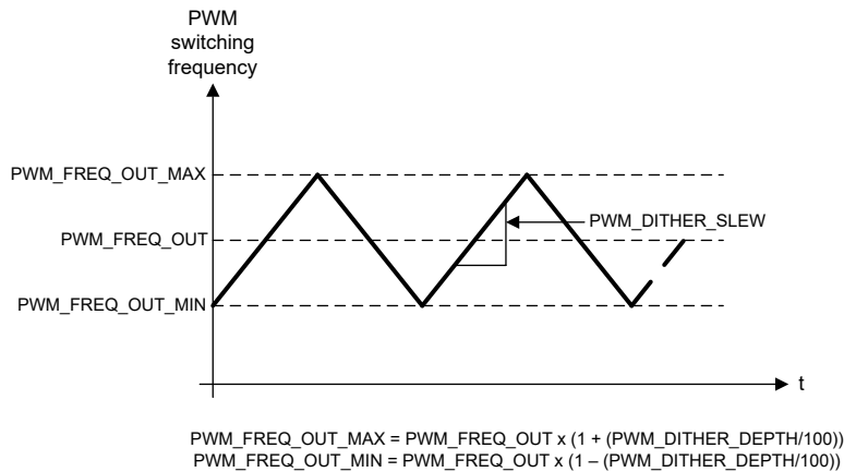
图 7-43. 三角 PWM 抖动
