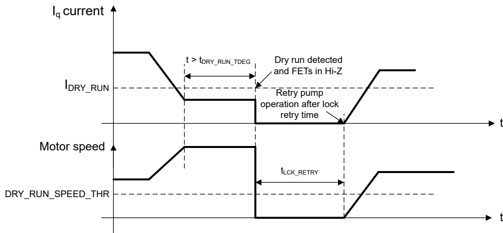
图 7-50. 空运行检测
