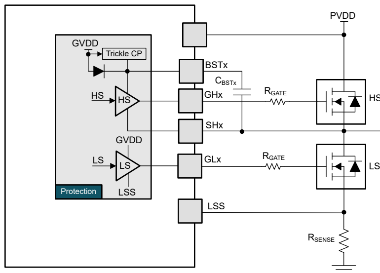
图 10-2. 具有串联电阻器的栅极驱动器输出
