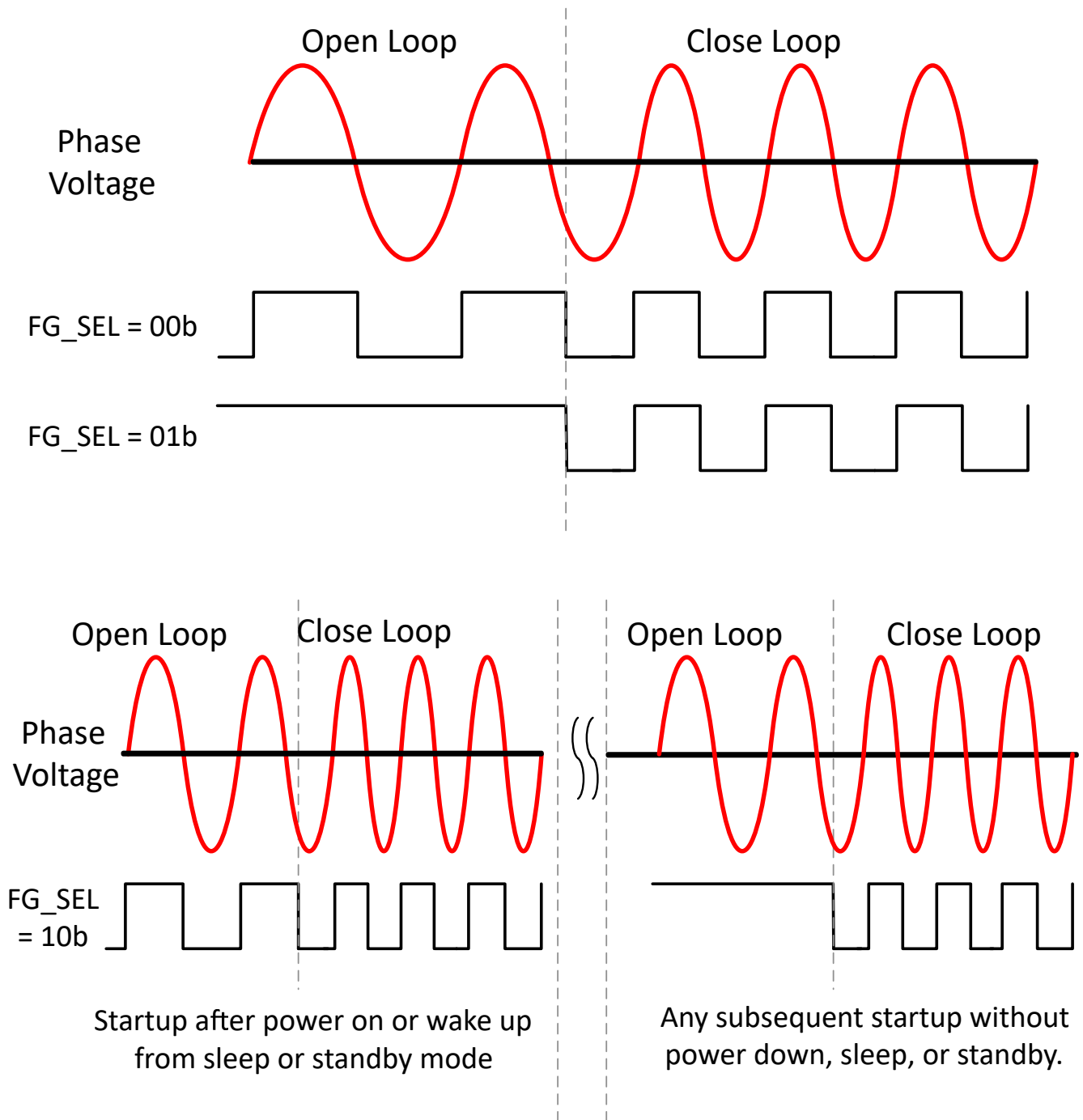
图 7-47. 开环期间的 FG 行为
