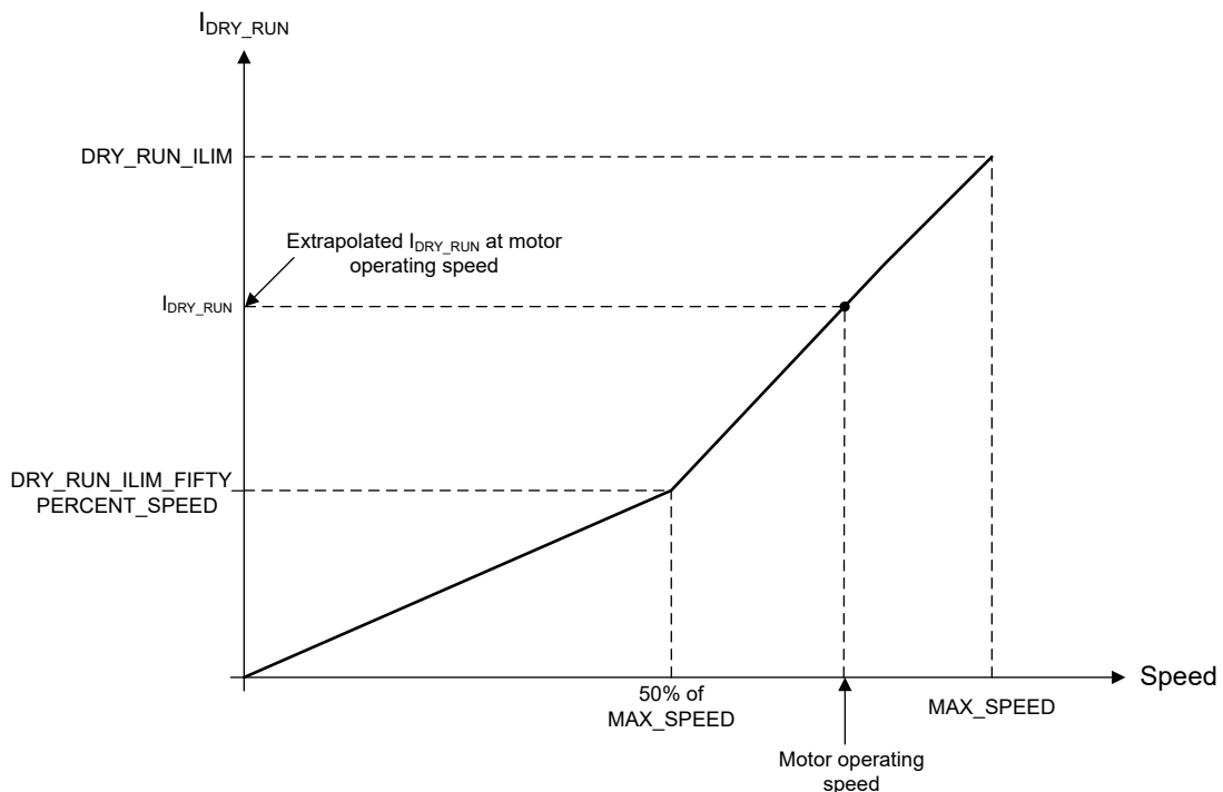
图 7-51. 用于空运行检测的可变电流阈值 ( I_{DRY\_RUN} )
