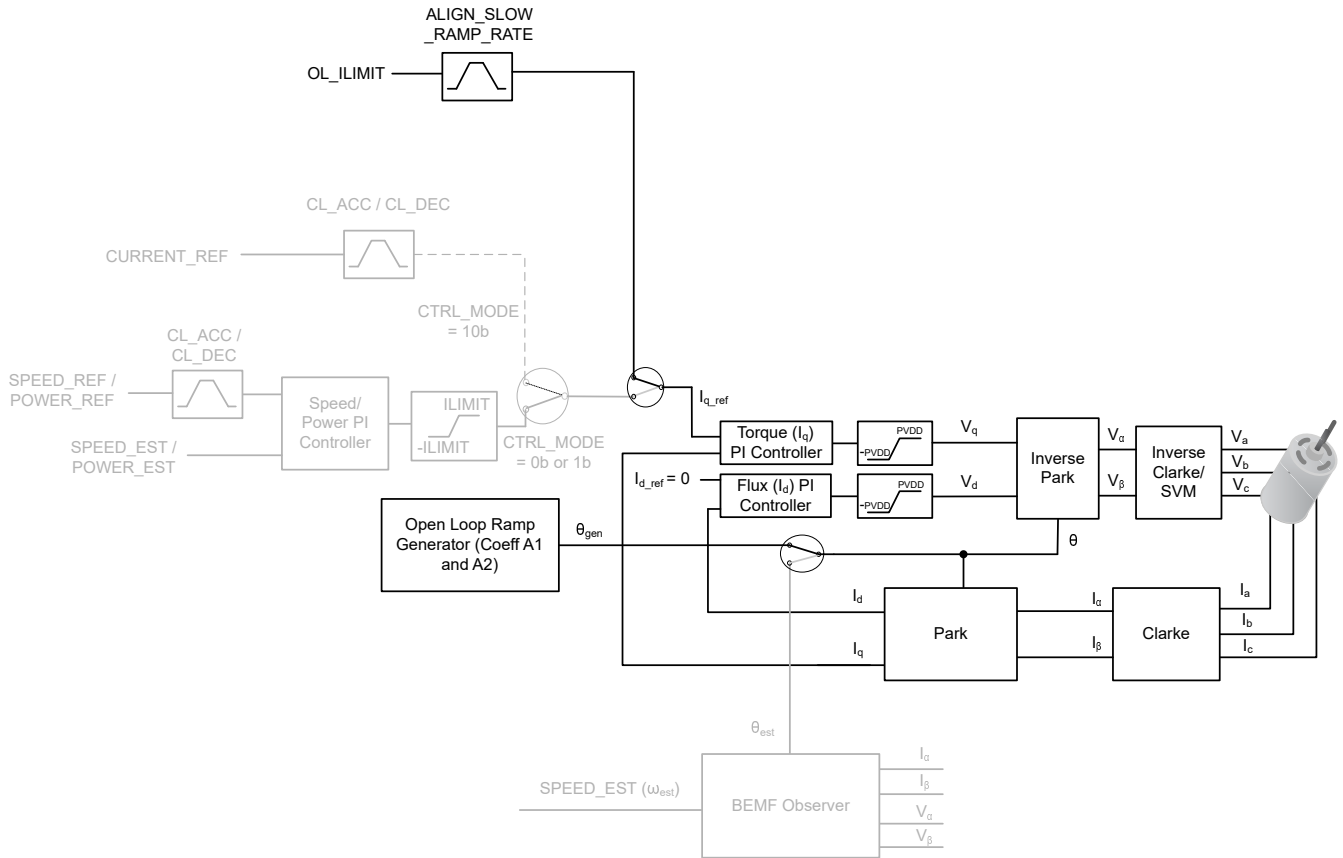
图 7-27. 开环
