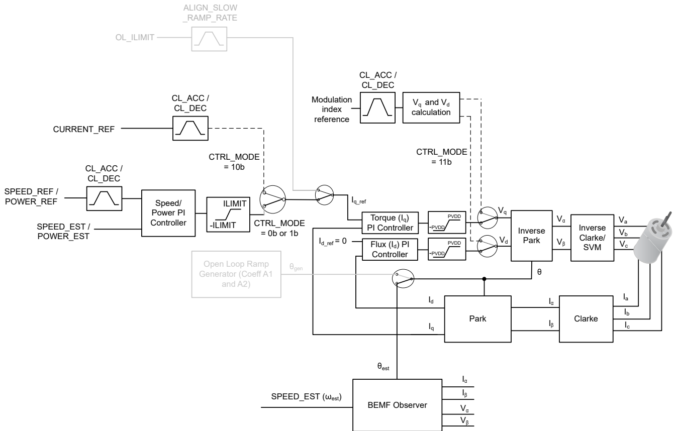
图 7-29. 开环到闭环转换
