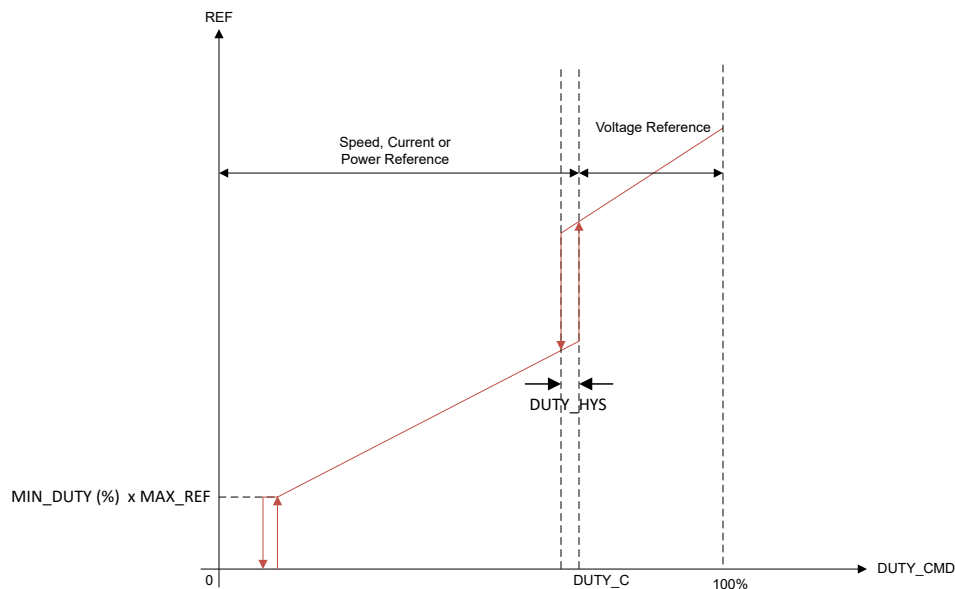
图 7-14. 多基准模式运行 (当 MIXED_MODE_CONFIG = 01b 时)
