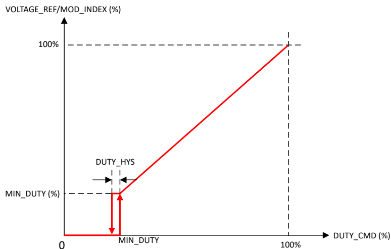
图 7-18. 电压基准传递函数
