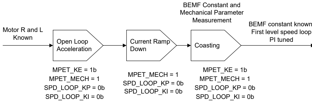
图 7-41. MPET 序列
