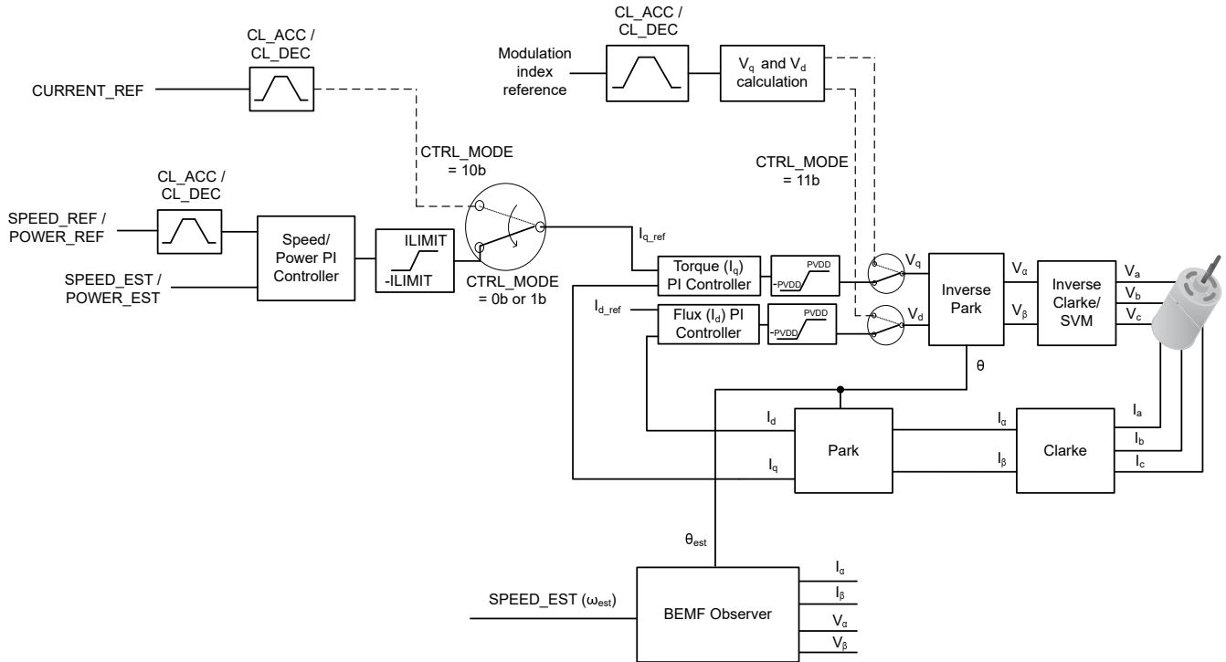
图 7-30. 闭环 FOC 控制
