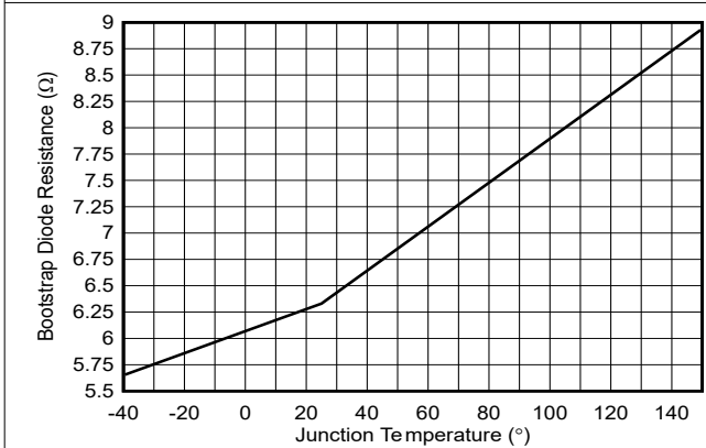
图 6-3. 自举二极管电阻与结温之间的关系
