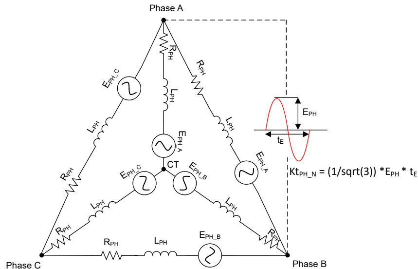
图 7-40. 电机反电动势常数
