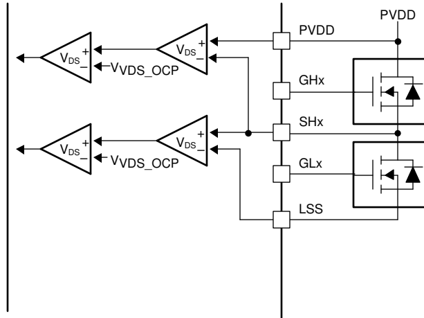
图 7-49. VDS 监控器
