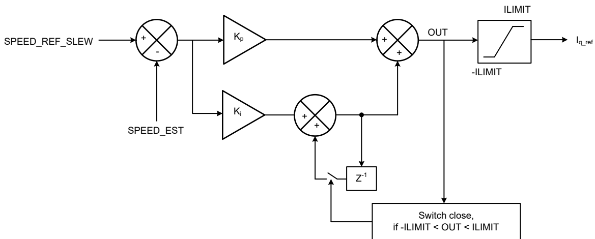
图 7-32. 速度 PI 控制
