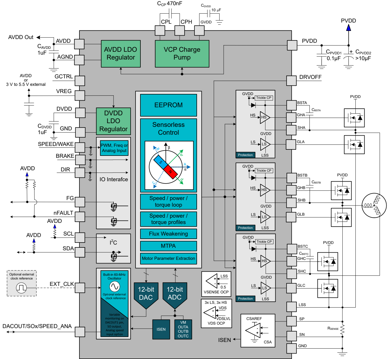
图 10-1. MCF8329HS 的典型原理图
