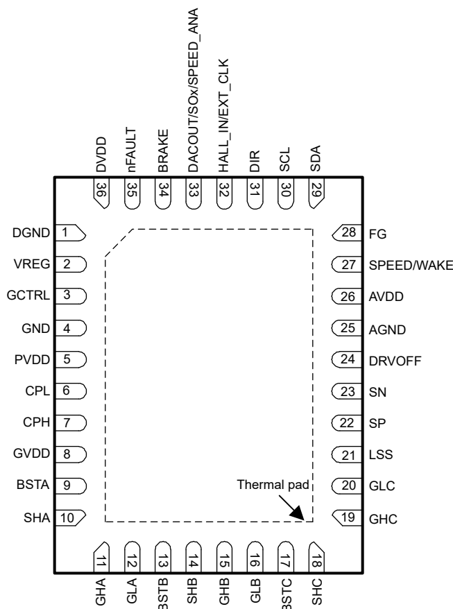
图 5-1. MCF8329HS 36 引脚 WQFN (带有外露散热焊盘) 顶视图
