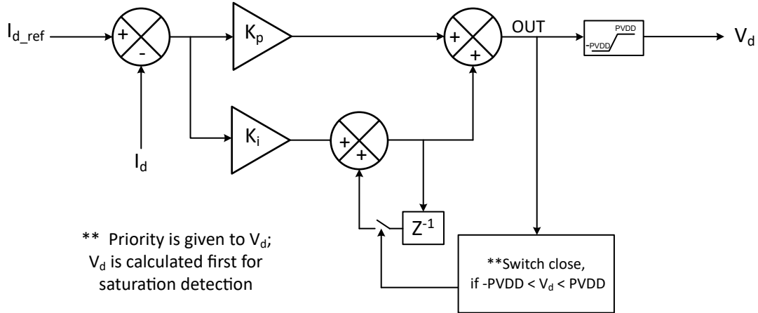
图 7-33. I_d 电流 PI 控制
