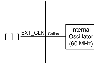
图 7-54. 外部时钟基准
