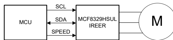
图 10-5. 采用 MCF8329HSULIREER 的 IEC 60730 功能安全系统
