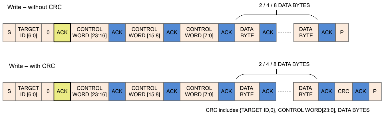
图 7-55. I 2 C 写入事务序列
