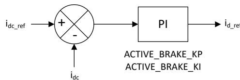
图 7-42. i_{d\_ref} 的主动制动电流控制环路
