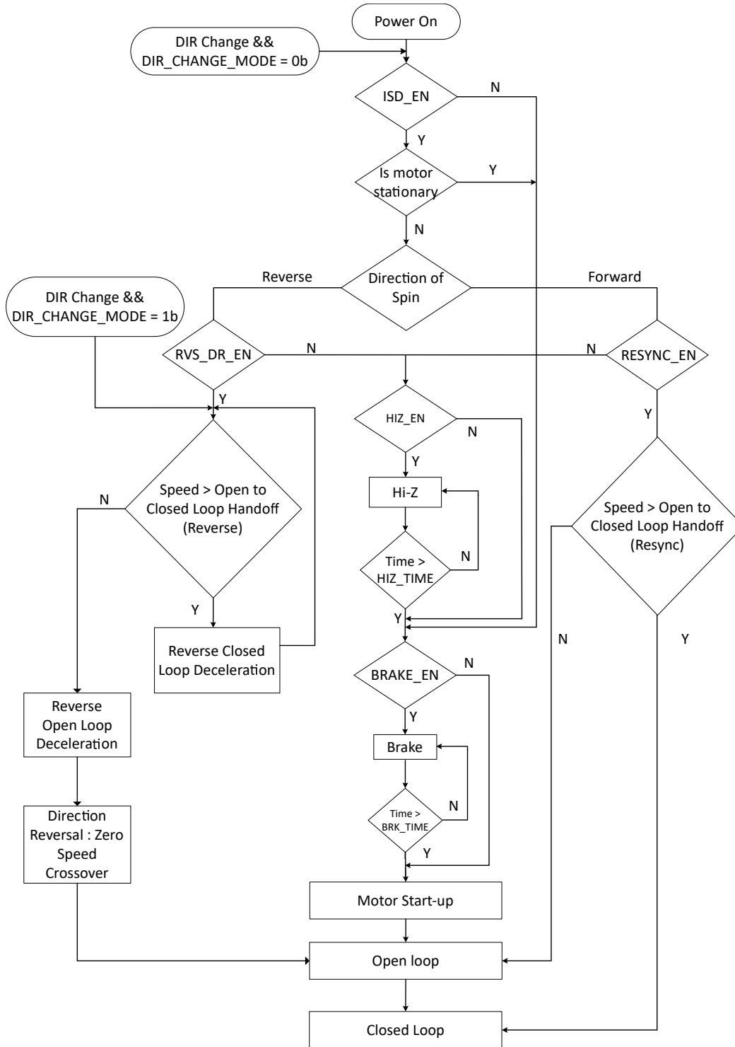
图 7-22. 电机启动流程
