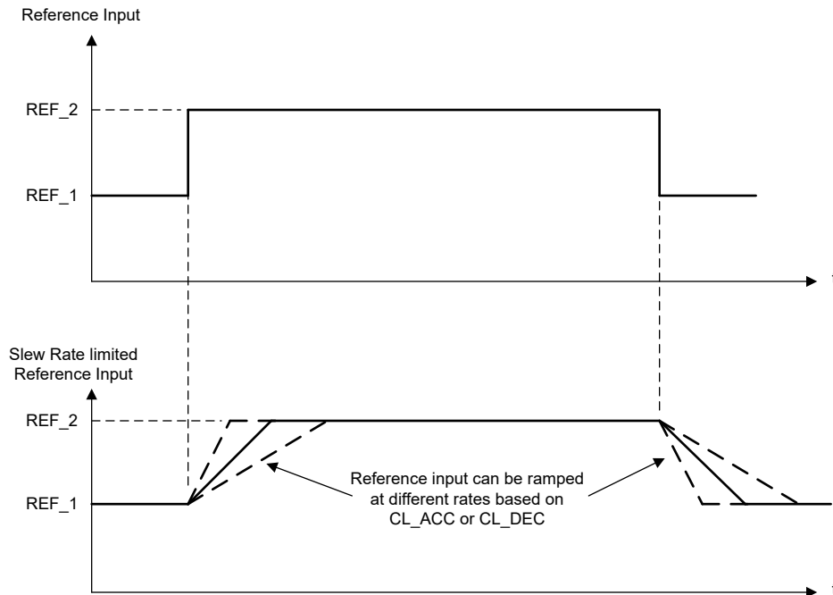
图 7-31. 闭环加速/减速压摆率
