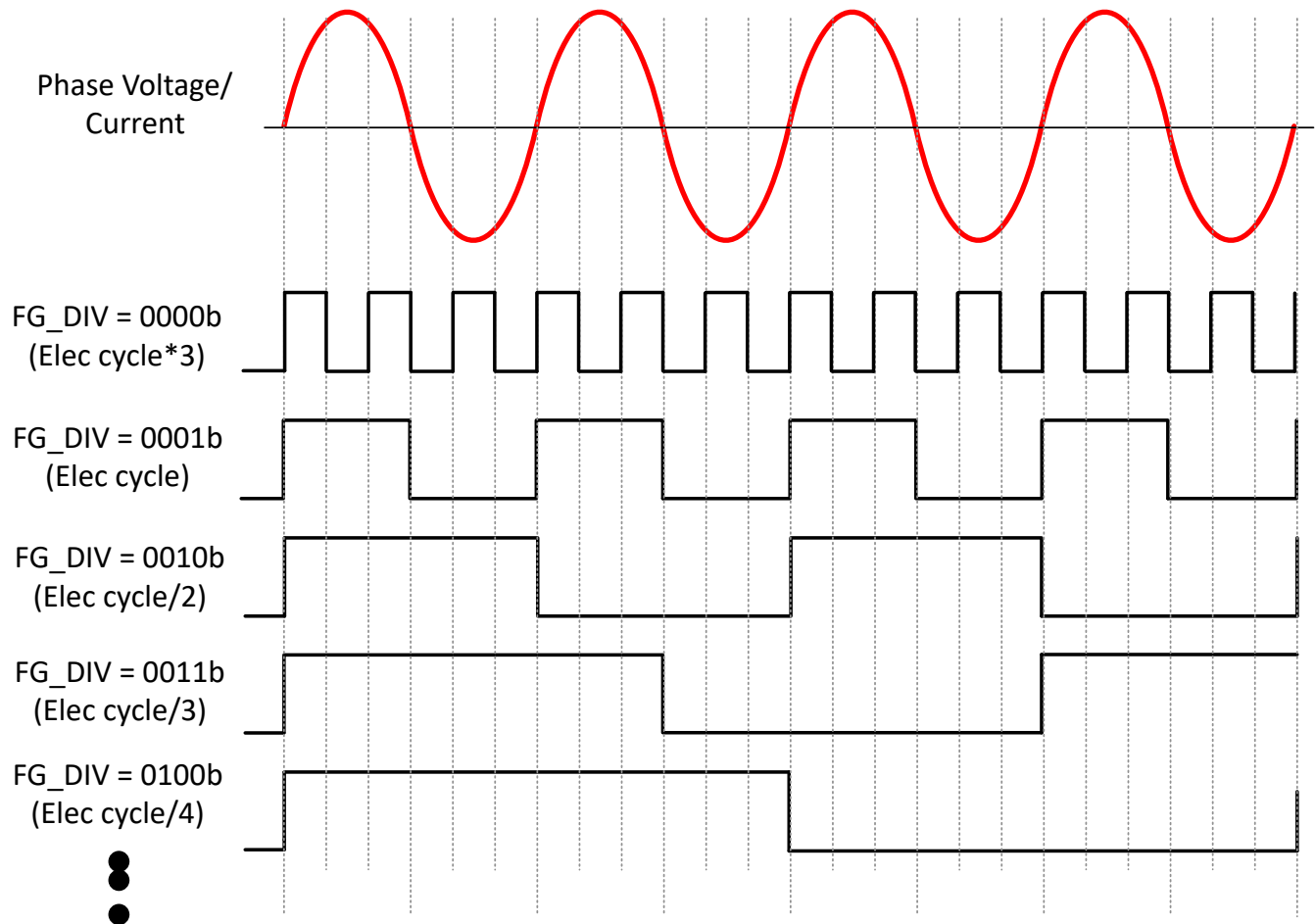
图 7-46. FG 分频器
