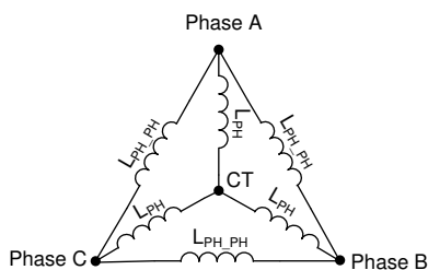
图 7-39. 电机电感
