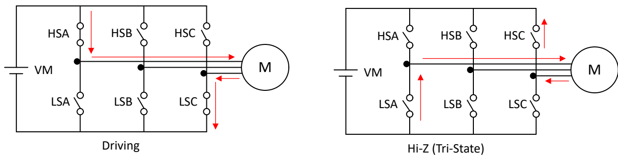
图 7-25. IPD 释放高阻态模式
