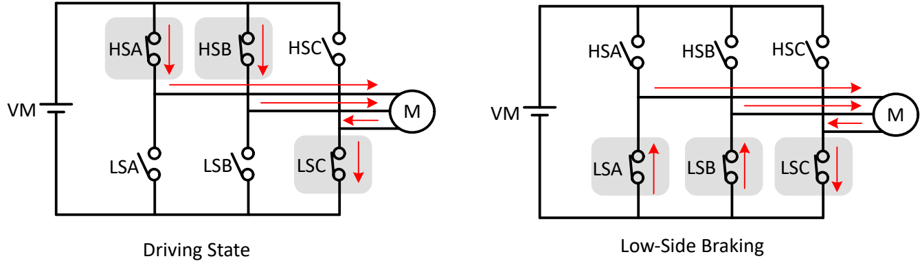
图 7-45. 低侧制动
