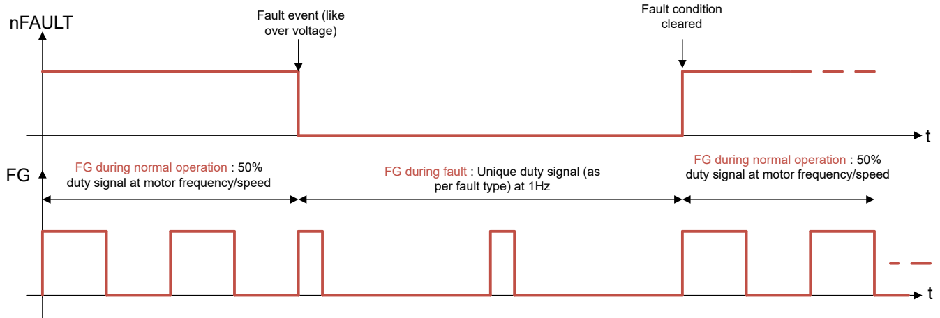
图 7-48. 通过 FG 进行故障指示
