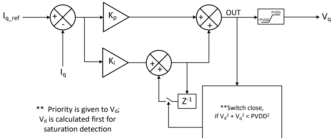
图 7-34. I_q 电流 PI 控制
