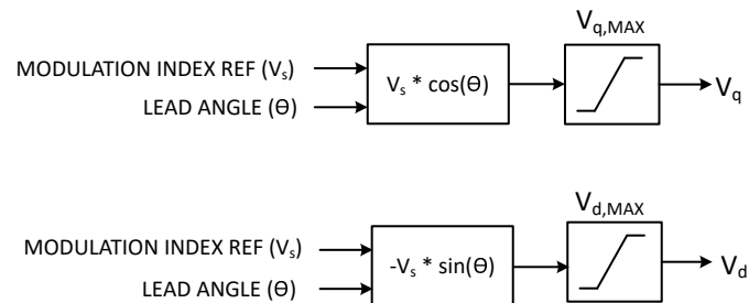
图 7-36. 开环电压控制
