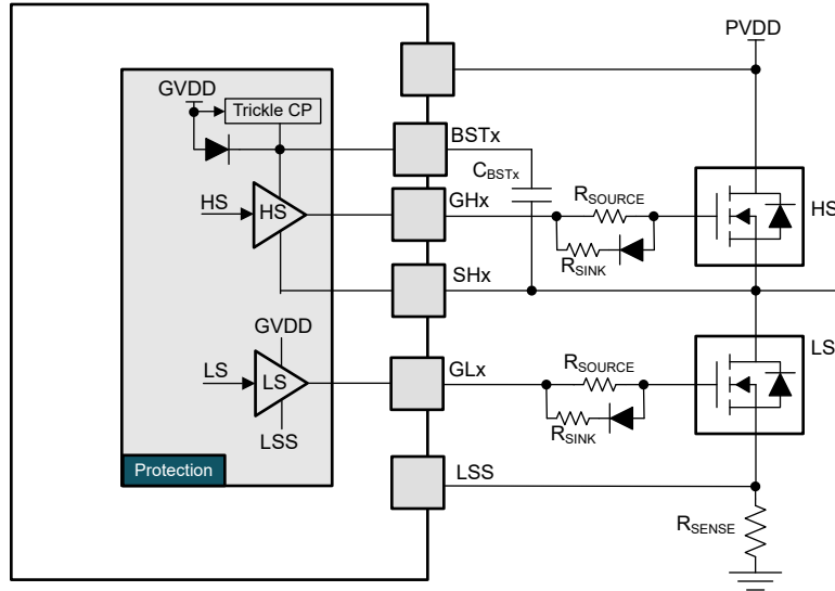
图 10-3. 具有独立拉电流路径和灌电流路径的栅极驱动器输出
