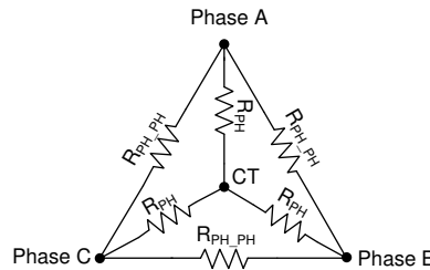
图 7-38. 电机电阻
