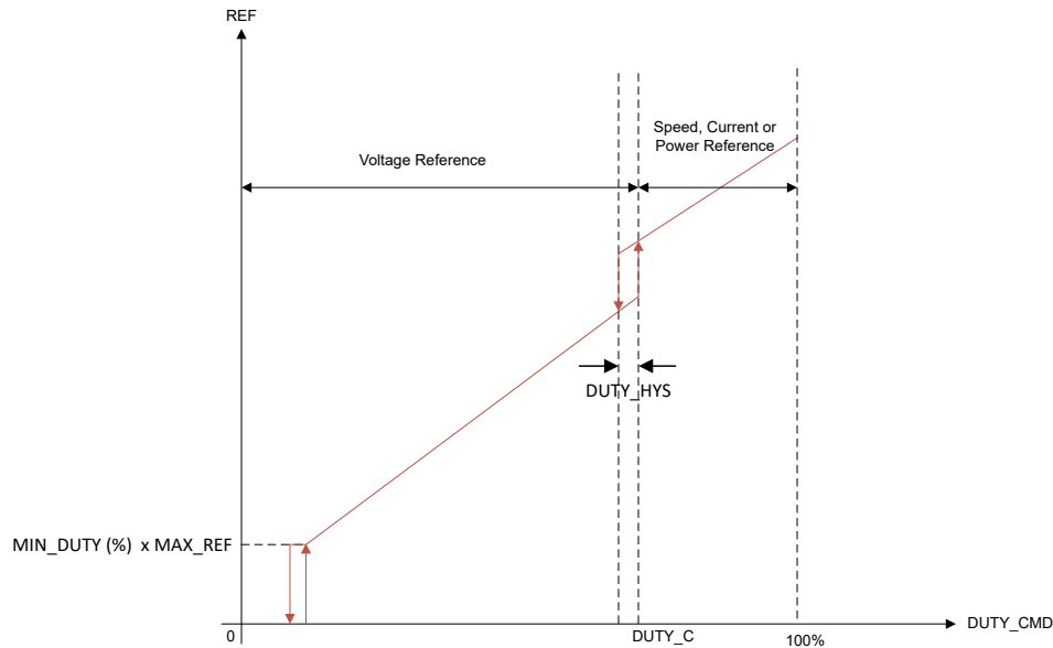
图 7-15. 多基准模式运行 (当 MIXED_MODE_CONFIG = 10b 时)
