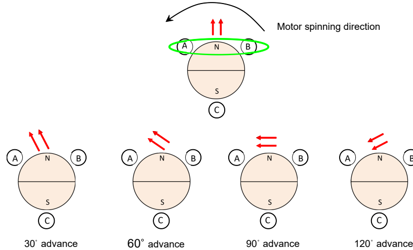
图 7-26. IPD 超前角度
