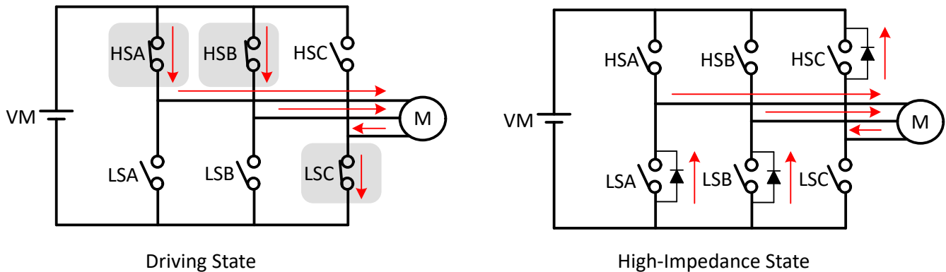
图 7-44. 滑行 (高阻态) 模式
