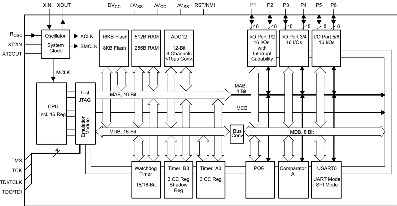
图 1-1. 功能方框图，MSP430F13x
