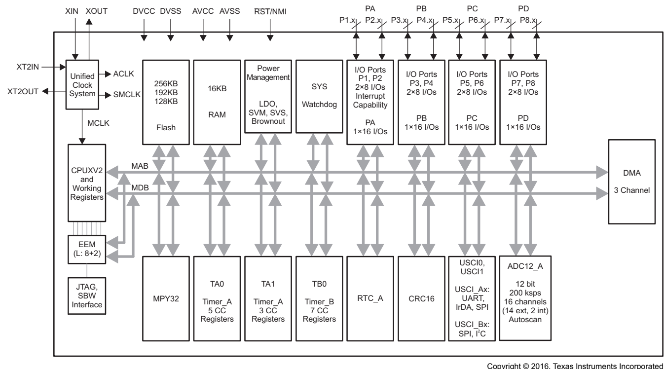
图 1-2. 功能方框图，MSP430F5437IPN、MSP430F5435IPN、MSP430F5418IPN
