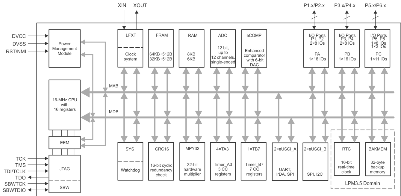
图 4-1. 功能模块图
