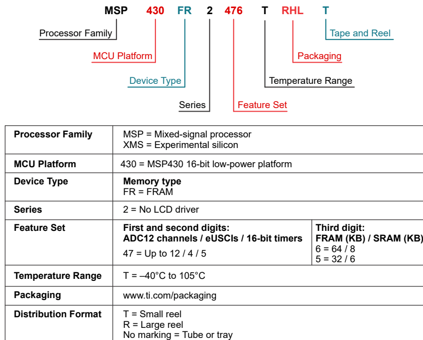
图 11-1. Device Nomenclature
