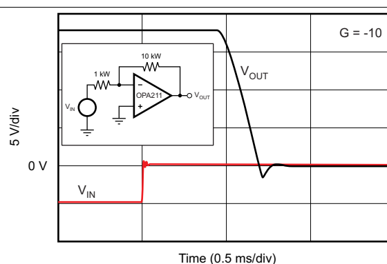
图 34. 大信号负极性建立时间
