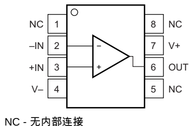
OPA211 D 封装 8 引脚 SOIC 俯视图
