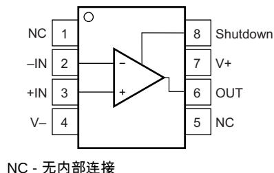
OPA211 DGK 封装 8 引脚 VSSOP 俯视图
