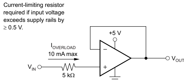
图 19. Input Current Protection
