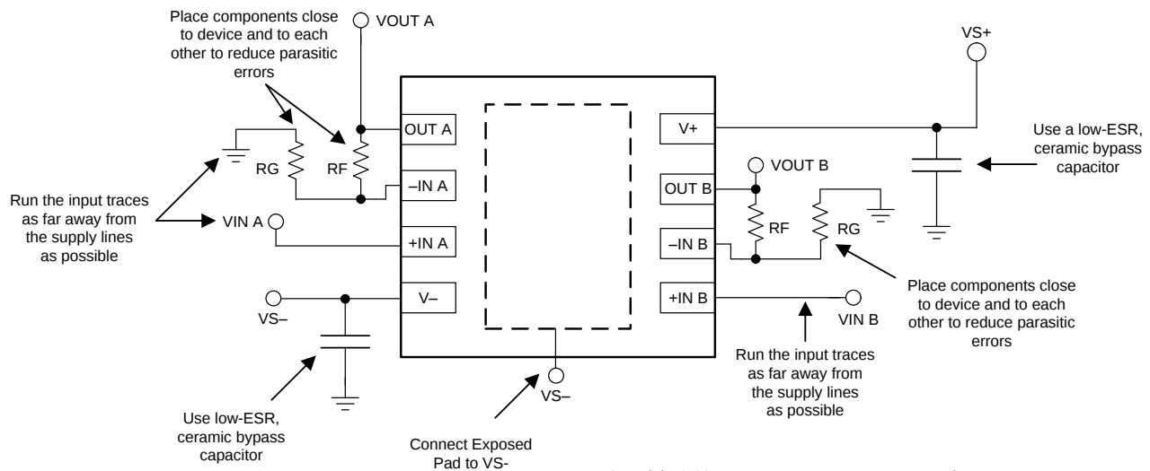
图 29. Layout Example
