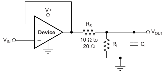
Figure 36. 改进电容负载驱动
