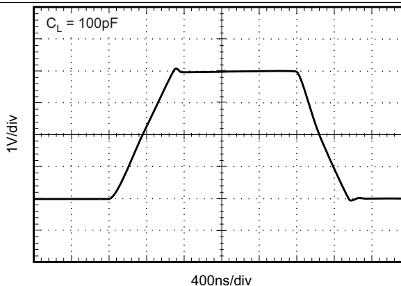
图 18. 大信号阶跃响应
