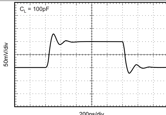
图 16. 小信号阶跃响应
