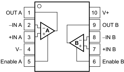
OPA2373: DRC 封装 10 引脚 VSSOP 俯视图
