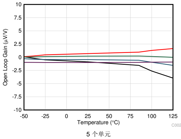
图 5-27. 开环增益与温度间的关系
