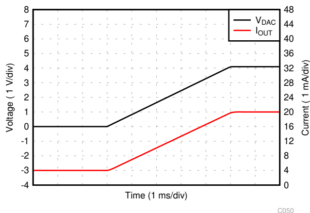
图 7-5. 4-20mA 环路响应
