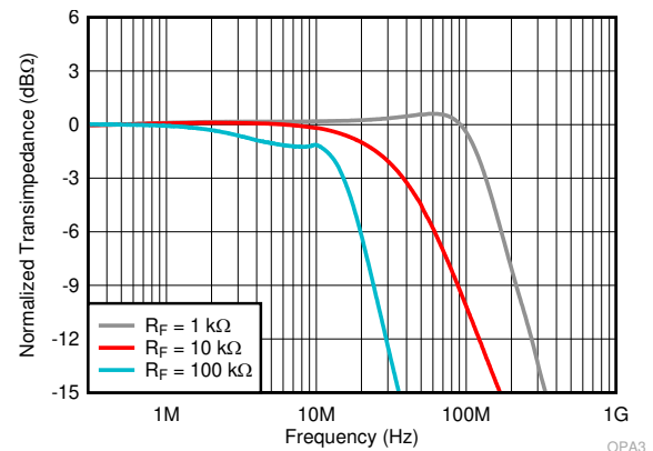
跨阻带宽与频率间的关系
