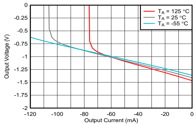
图 6-28. Output Swing vs Sinking Current
