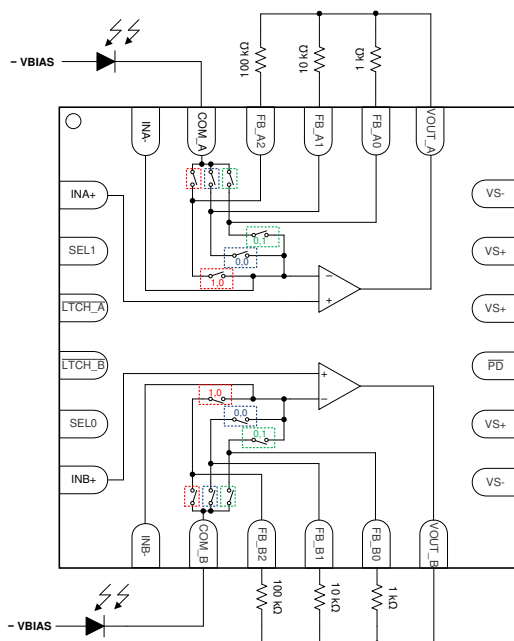
方框图
