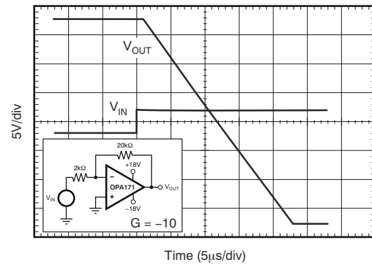
图 5-26. 正过载恢复
