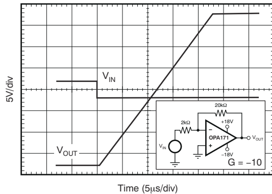
图 5-27. 负过载恢复
