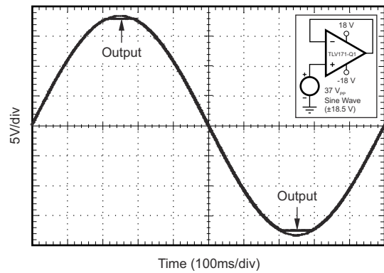
图 6-1. 无相位反转
