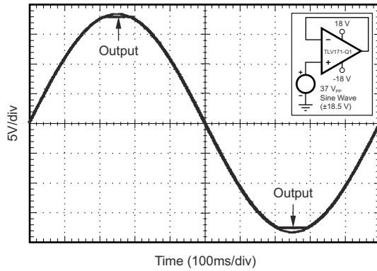
图 5-25. 无相位反转
