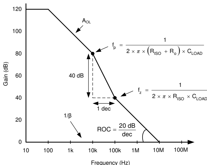
图 7-3. 具有 R_{ISO} 补偿的单位增益放大器
