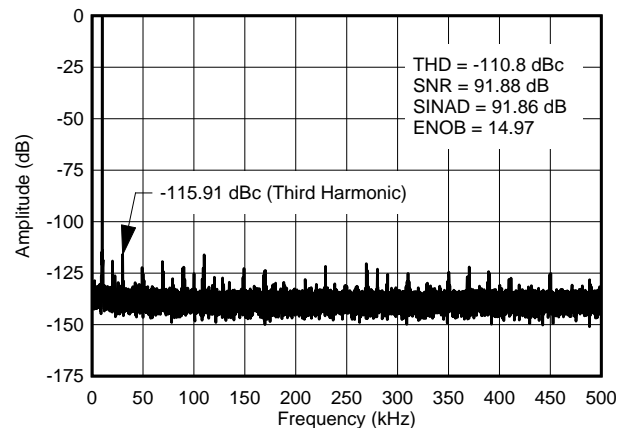
16 位 SAR ADC, f_{\text{IN}} = 10\text{kHz} , 1MSPS FFT
