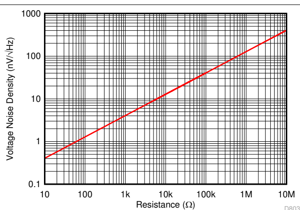
图 8-9. Thermal Noise Density vs Resistance
