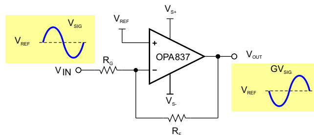
图 63. Inverting Amplifier
