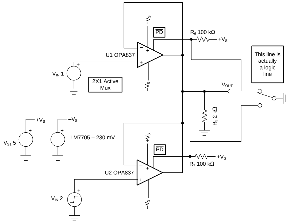
图 87. 2:1 Active Multiplexer
