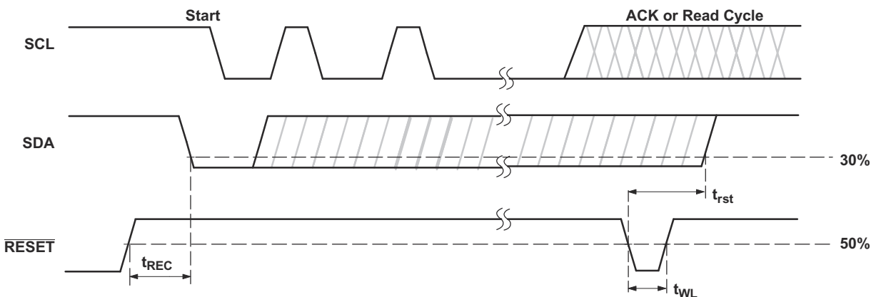
图 7-2. Reset Timing
