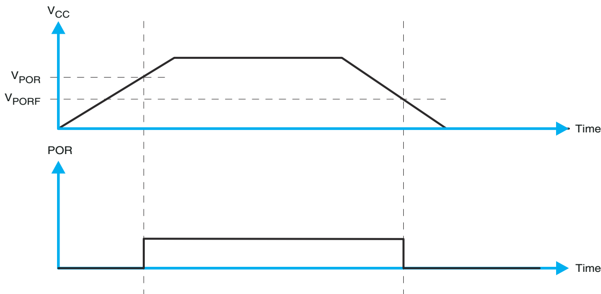
图 8-9. V_{POR}
