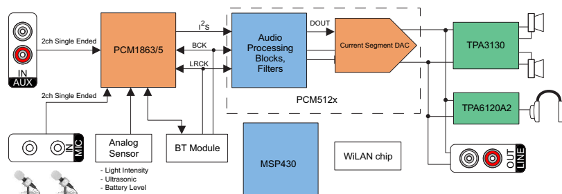
简化系统图
