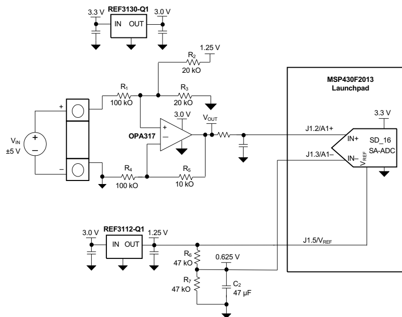
图 8-2. 适用于低功耗 ADC 的低功耗基准和双极电压调节电路
