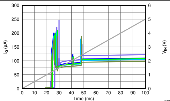
图 6-19. REF3125-Q1 启动
