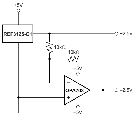
图 7-5. REF3125-Q1 与 OPA703 结合使用可产生正向和负向基准电压
