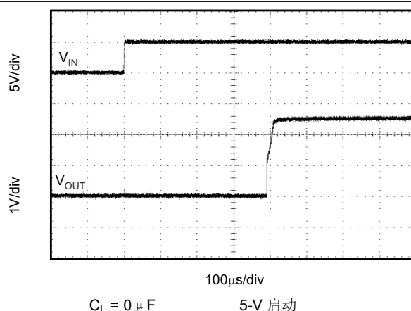
图 6-10. 阶跃响应
