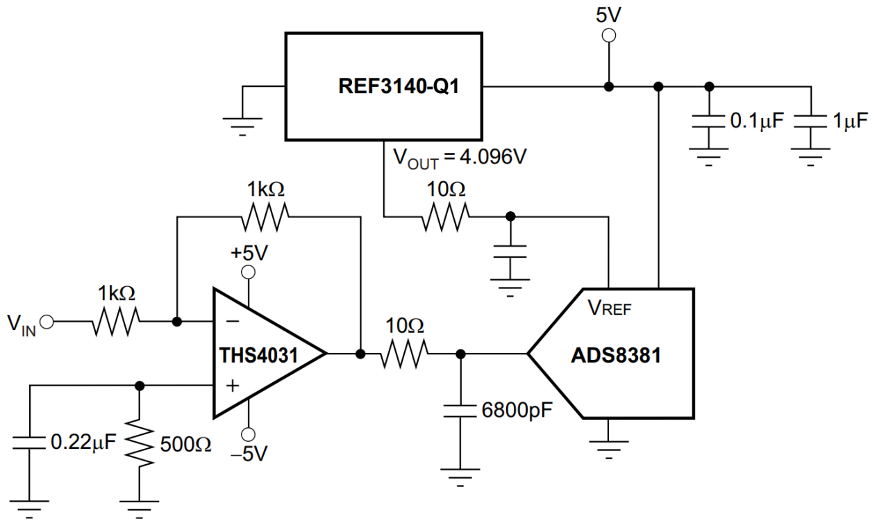
图 7-8. REF3140-Q1 为驱动 ADS8381 提供精确基准
