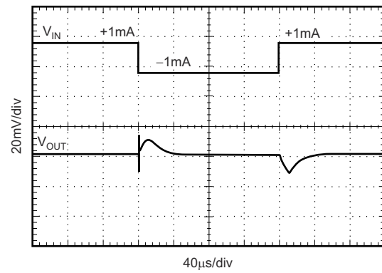
图 6-16. 负载瞬态
