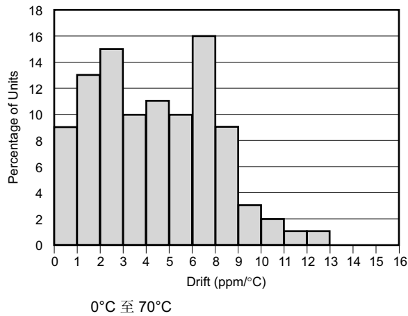
图 6-1. 温漂
