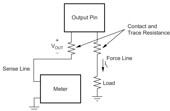
图 7-4. REF31xx-Q1 的准确负载调整
