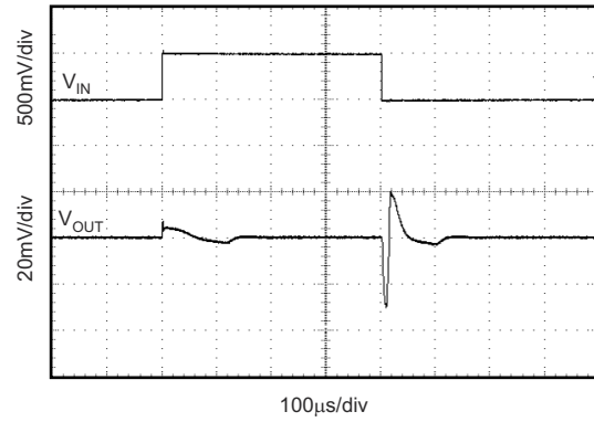
图 6-14. 线路瞬态
