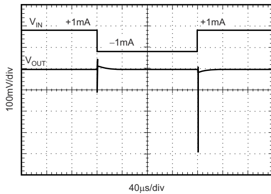
图 6-15. 负载瞬态
