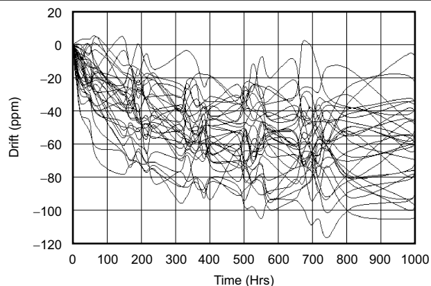
图 6-12. REF3112 长期稳定性
