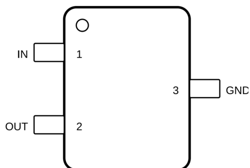
图 5-1. DBZ 封装 3 引脚 SOT-23 顶视图
