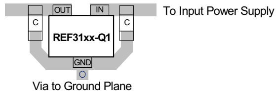
图 8-6. 布局示例
