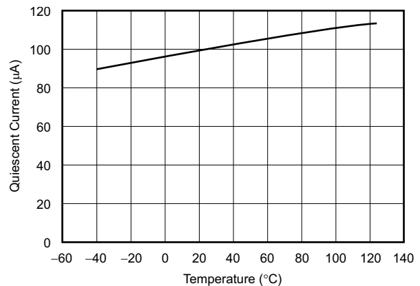
静态电流与温度间的关系
