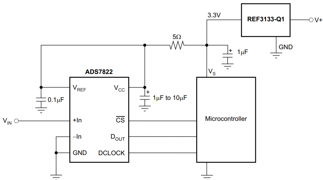
图 7-6. 基本数据采集系统 1
