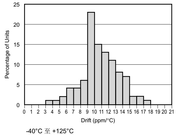
图 6-2. 温漂
