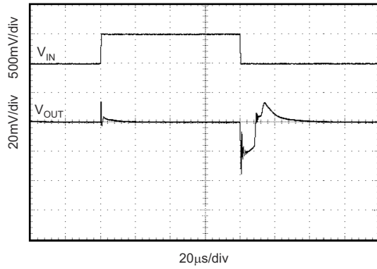
图 6-13. 线路瞬态
