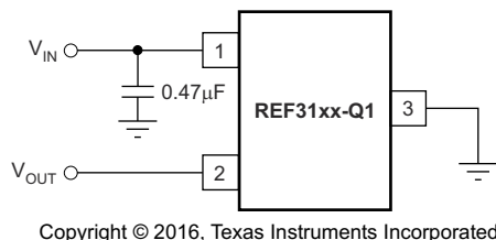
图 8-1. 运行 REF31xx-Q1 的典型连接
