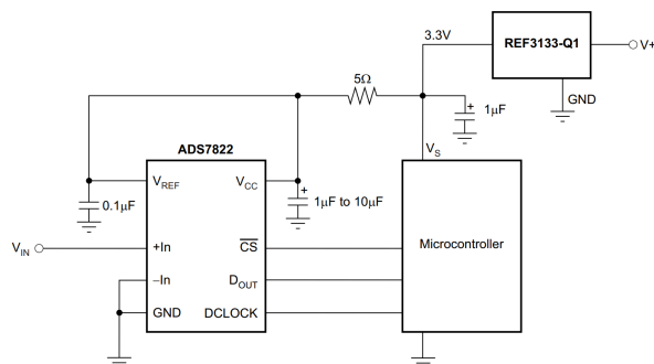
典型应用
