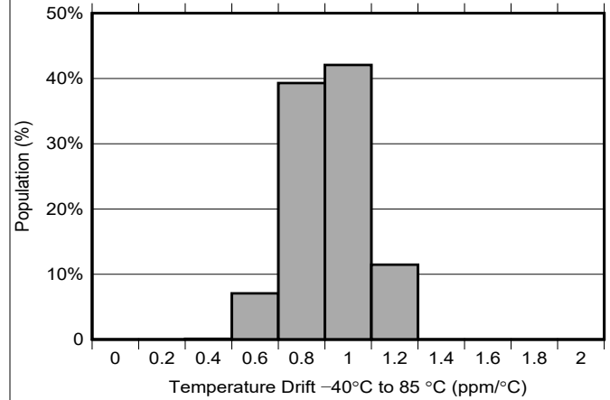
图 7-4. Temperature Drift Distribution (REF7012QDGKR)
