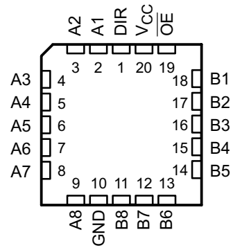
图 4-2. SN54AC245 FK Package Top View
