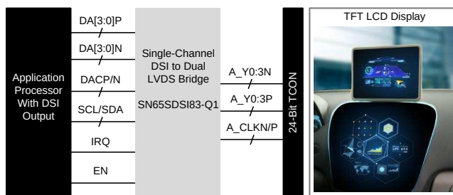
SN65DSI83-Q1 原理图
