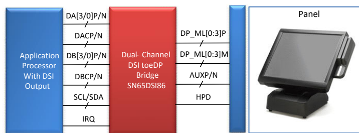
简单方框图
