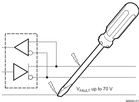
总线对电源短路的示例
