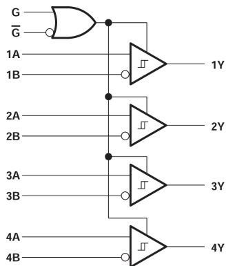
逻辑图
