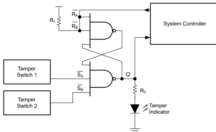
图 8-1. 典型应用框图
