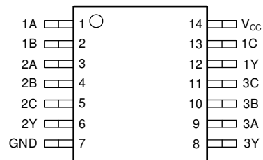
图 4-4. SN74AC10 D、DB、N、NS 或 PW 封装 (顶视图)
