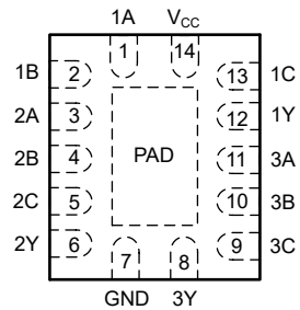
图 4-3. SN74AC10 BQA 封装 (顶视图)
