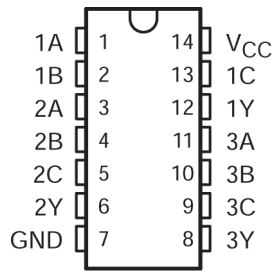
图 4-1. SN54AC10 J 或 W 封装 (顶视图)
