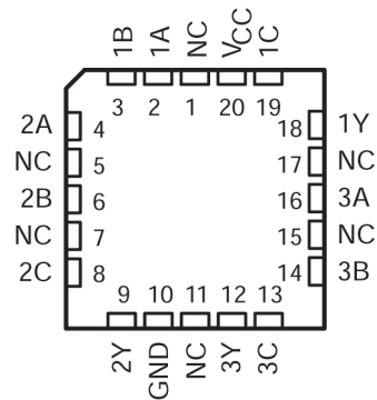
图 4-2. SN54AC10 FK 封装 (顶视图)
