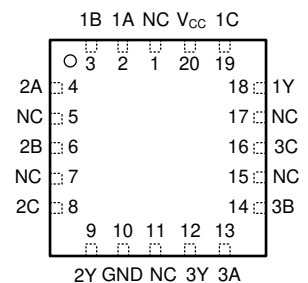
图 4-2. FK 封装 (顶视图)
