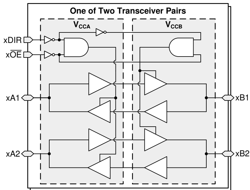
功能方框图
