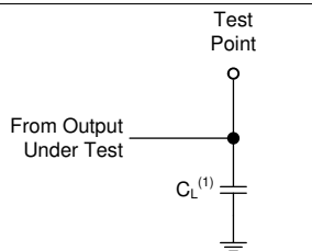
图 5. Load Circuit
