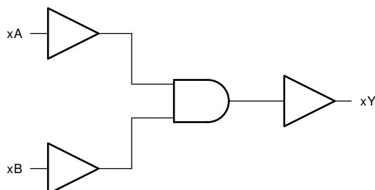
图 6-1. 功能方框图
