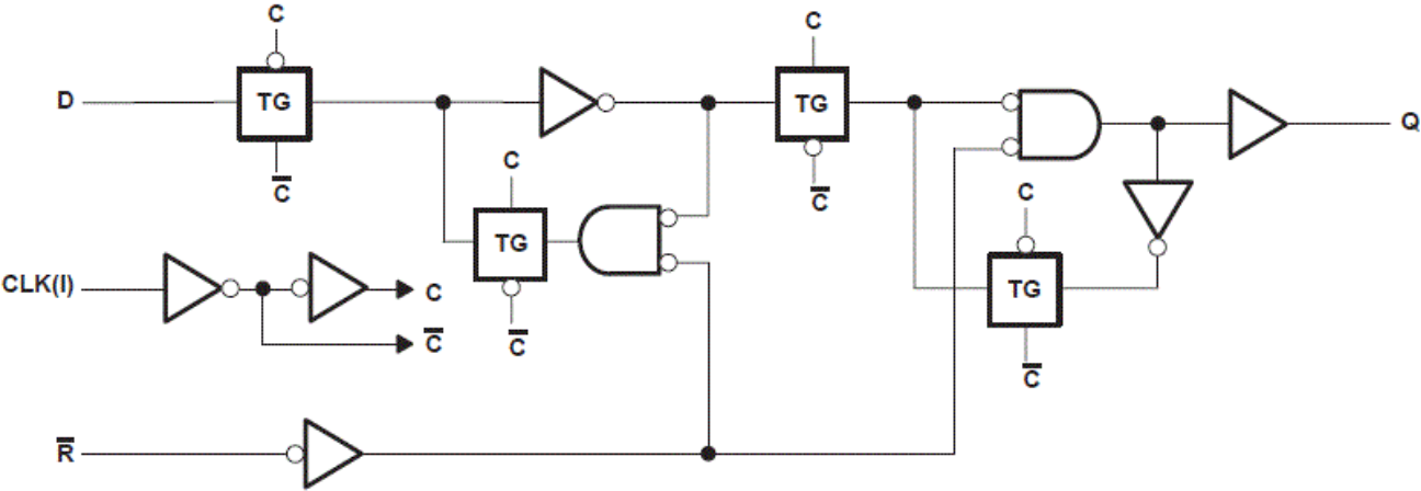
图 7-2. 展示各触发器的逻辑图 (正逻辑)
