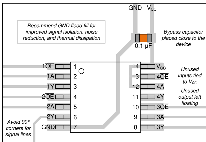
图 8-4. SN74LVC125A 的示例布局
