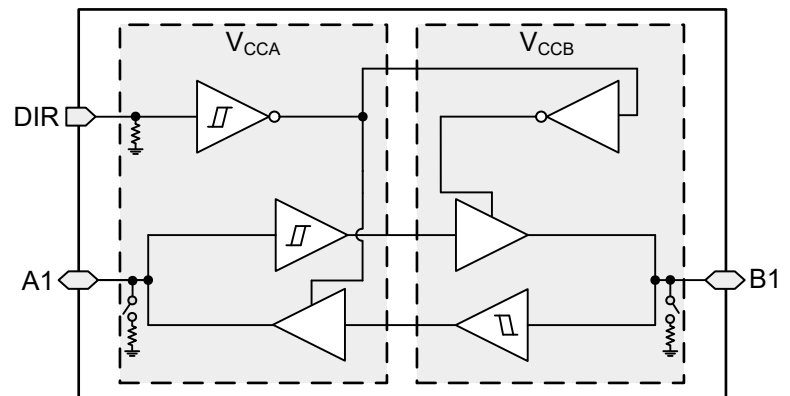
SN74LXC1T45 框图
