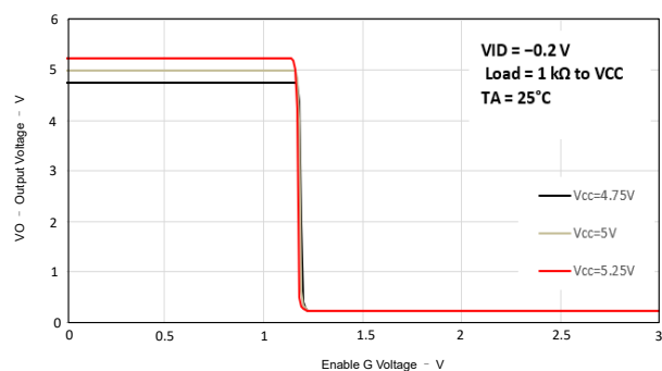
图 5-7. Output Voltage vs Enable G Voltage
