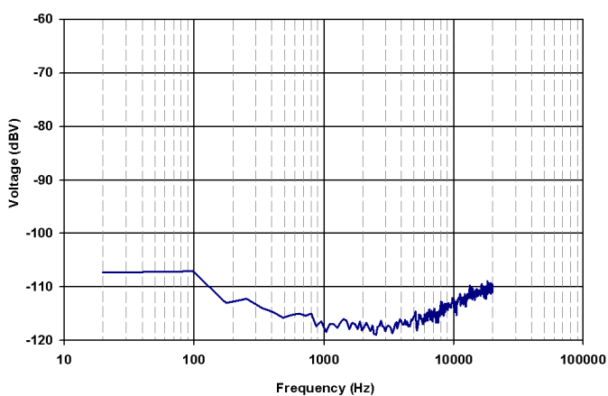
NOISE FFT
