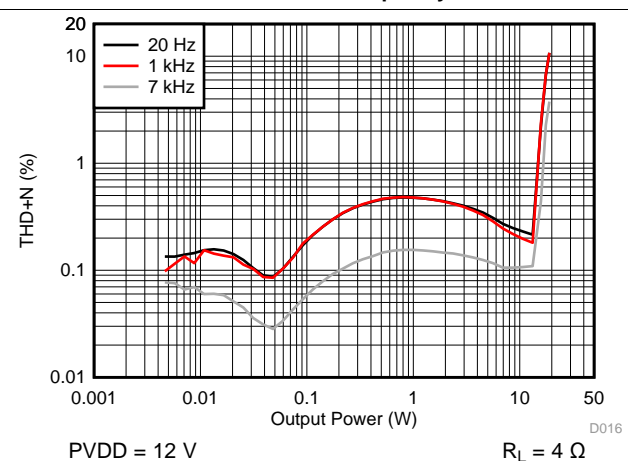
图 20. THD+N vs Output Power - PBTL
