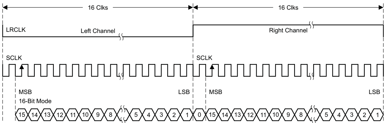
图 57. I 2 S 32-f s Format
