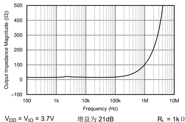
图 6-3. PGA Z_{OUT} 与频率之间的关系
