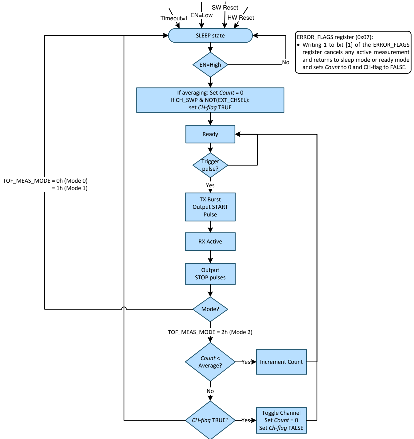
图 8-14. 简化的 TDC1000-Q1 状态机图
