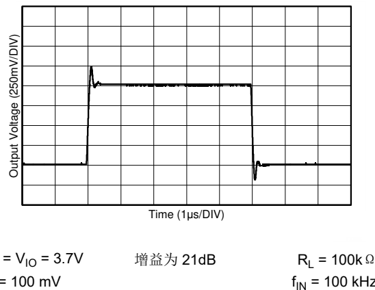
图 6-7. PGA 响应
