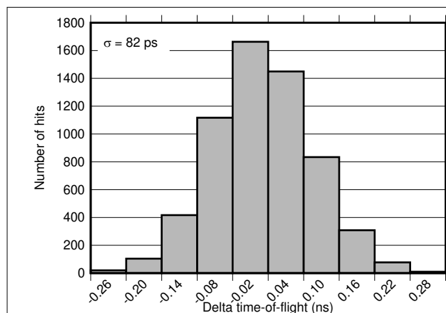
图 9-10. 原始校准数据直方图
