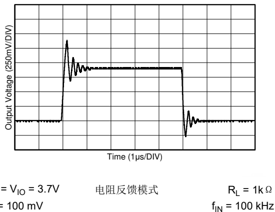
图 6-6. LNA 响应
