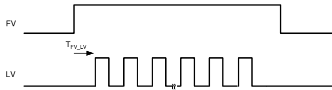
图 7-5. Minimum FV to LV
