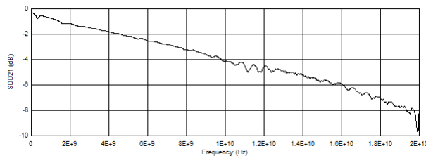
图 9-5. Post-Channel Insertion Loss at TTP4
