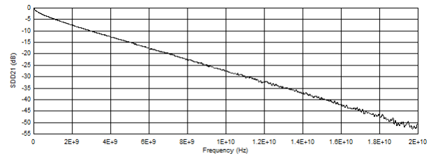
图 9-4. Pre-Channel Insertion Loss at TTP2
