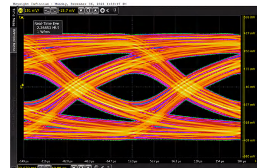
图 9-8. 5.94 Gbps Input Eye at TTP2 After Pre-Channel
