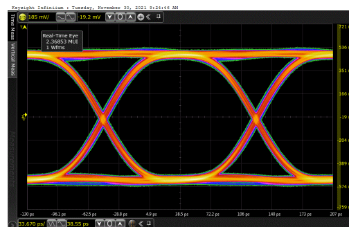
图 9-9. 5.94 Gbps Output Eye at TTP4 After Pre and Post Channels
