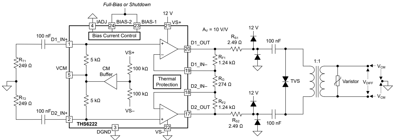
图 6-7. Surge Test Configuration
