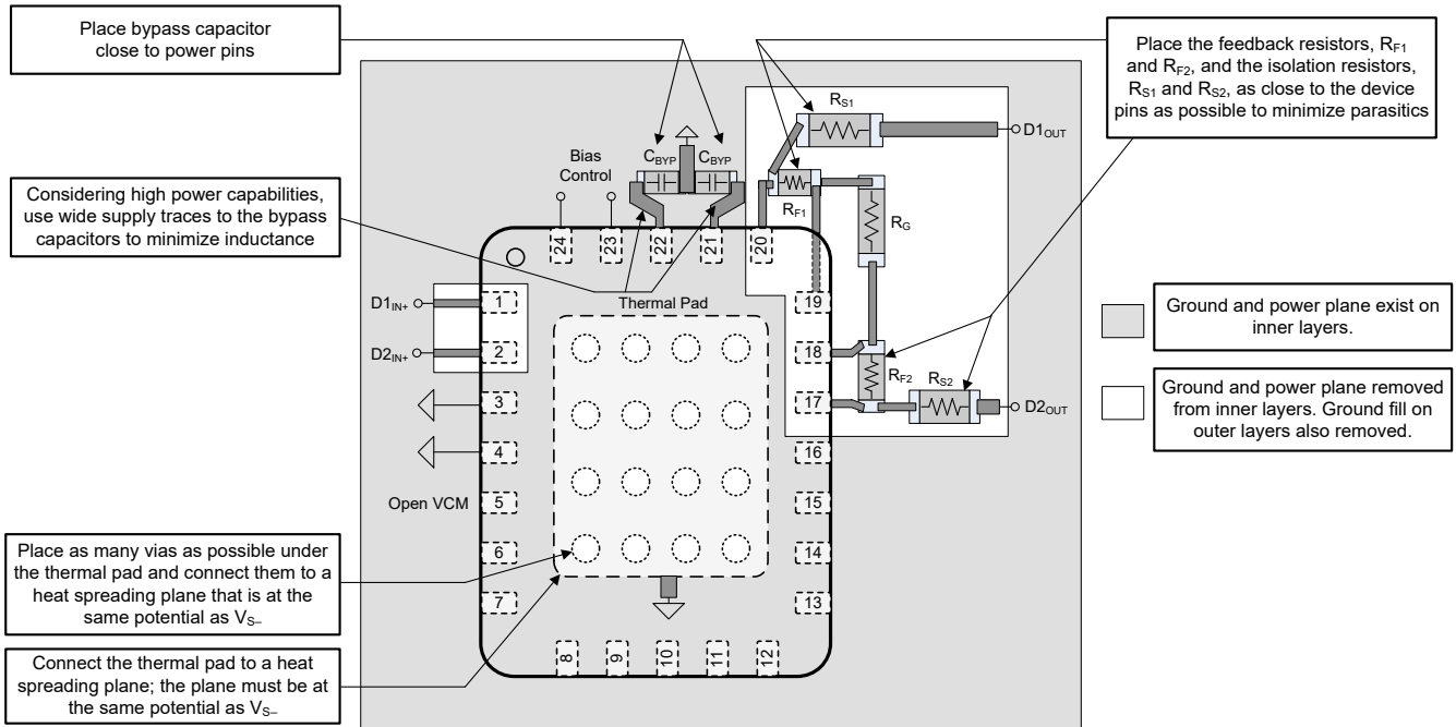
图 7-6. Layout Recommendations
