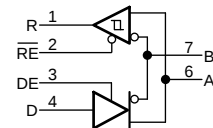
THVD1551 简化原理图
