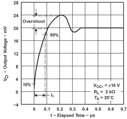
图 5-56. 输出电压与经历时间的关系
