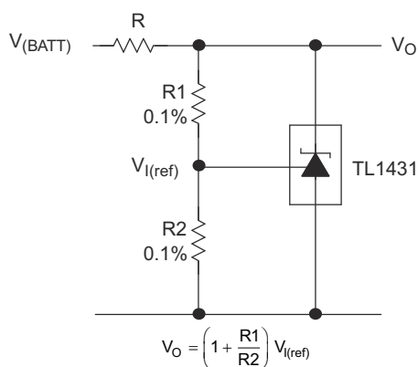
图 8-3. 并联稳压器
