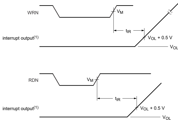
图 4-7. Port Timing
