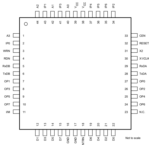
图 3-1. 80xxx Mode FR (QFP) Package (Top View)
