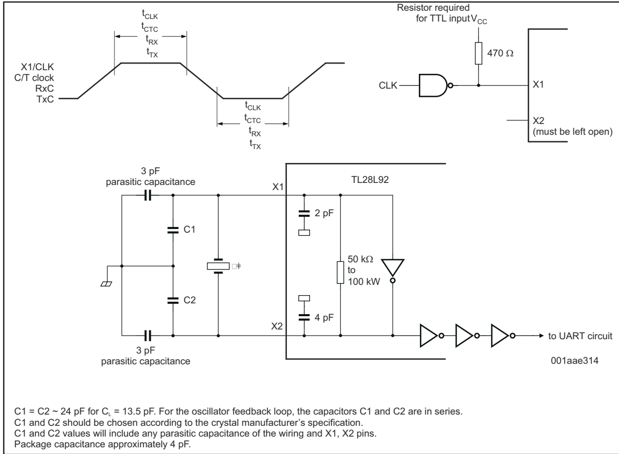
图 4-9. Clock Timing
