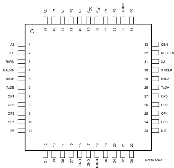
图 3-2. 68xxx Mode FR (QFP) Package (Top View)
