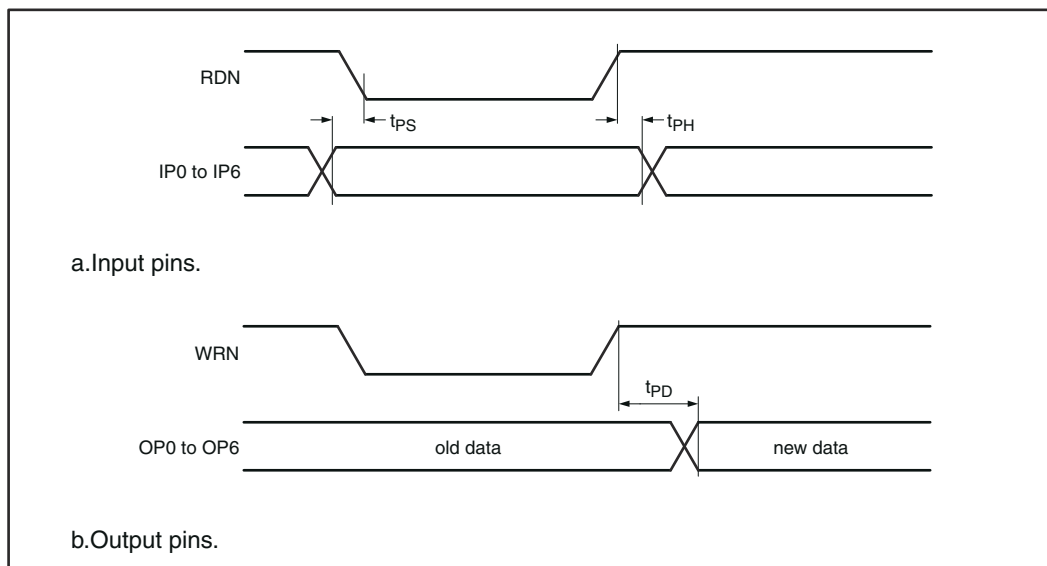
图 4-7. Port Timing
