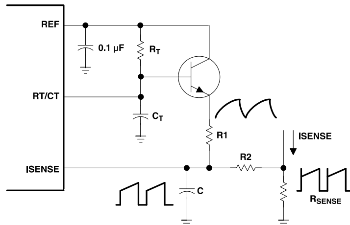
图 6-2. Slope Compensation
