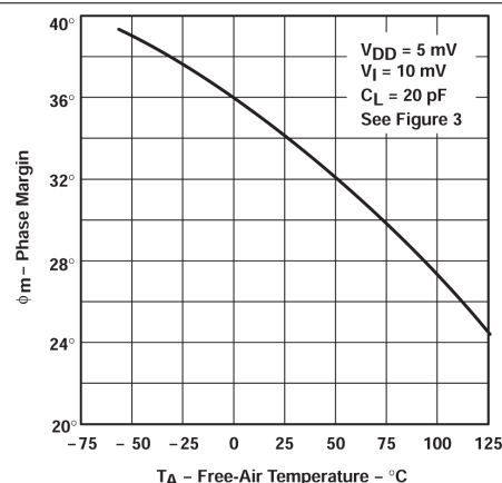
图 5-28. 相位裕度与自然通风温度间的关系
