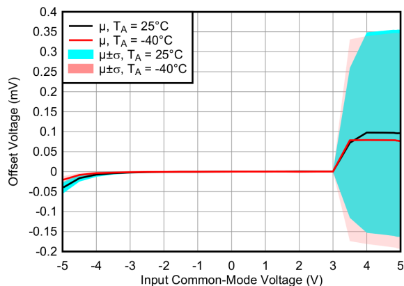
图 7-3. 偏移电压与输入共模电压间的关系
