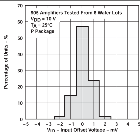
图 5-2. TLC27L2 输入失调电压的分布
