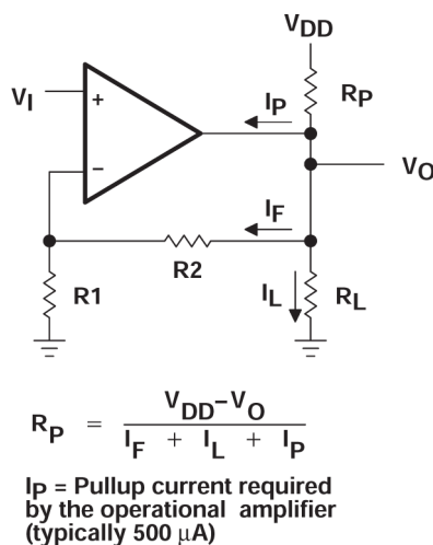
图 7-8. 使用阻性上拉来提高 V_{OH}
