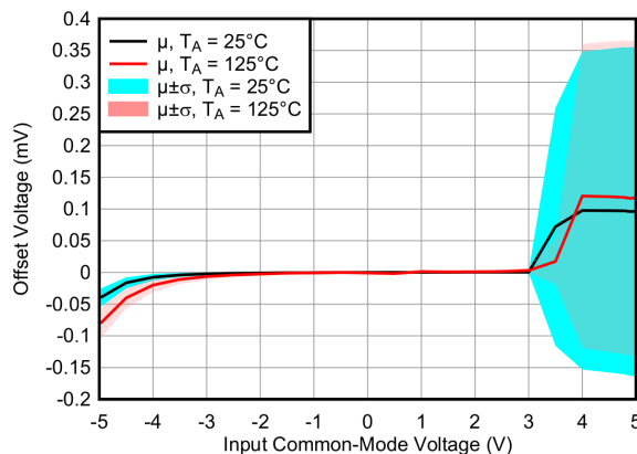
图 7-4. 偏移电压与输入共模电压间的关系
