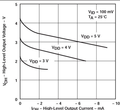
图 5-5. 高电平输出电压与高电平输出电流间的关系
