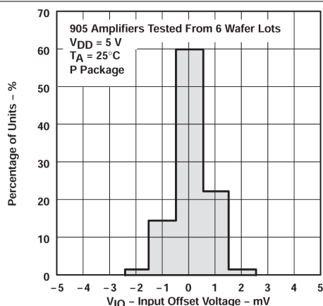
图 5-1. TLC27L2 输入失调电压的分布
