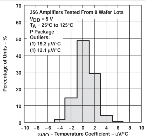
图 5-3. TLC27L2C 与 TLC27L7 输入偏移电压温度系数的分布
